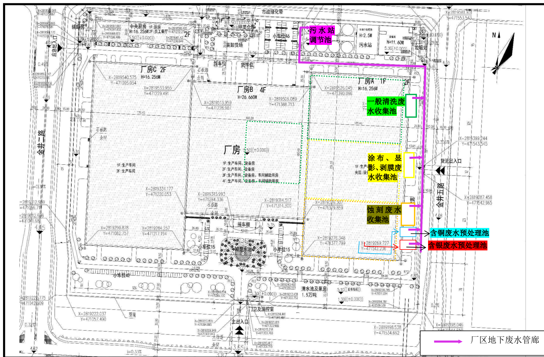
附图 16 生产废水分类收集线路图
