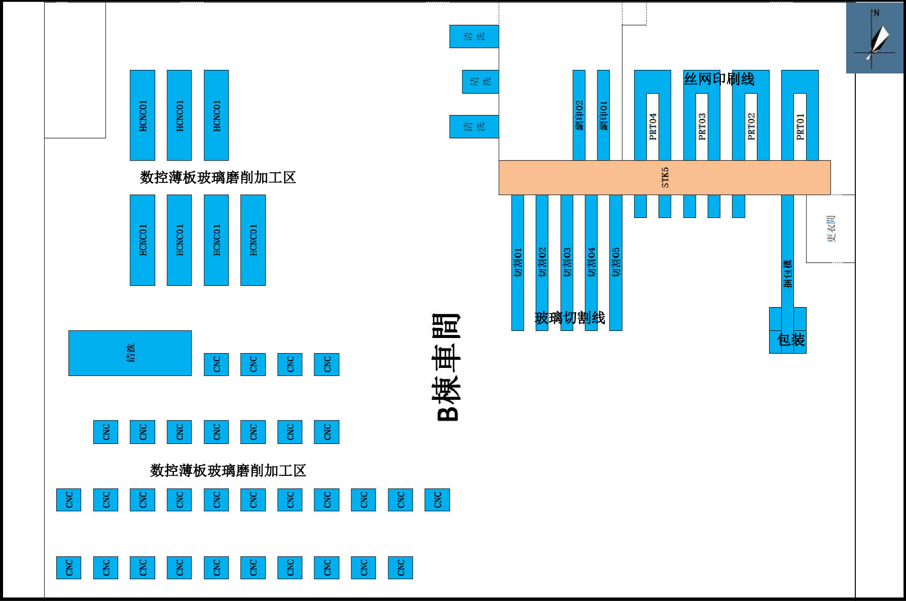
附图 5 车间平面布置图（厂房 B）
