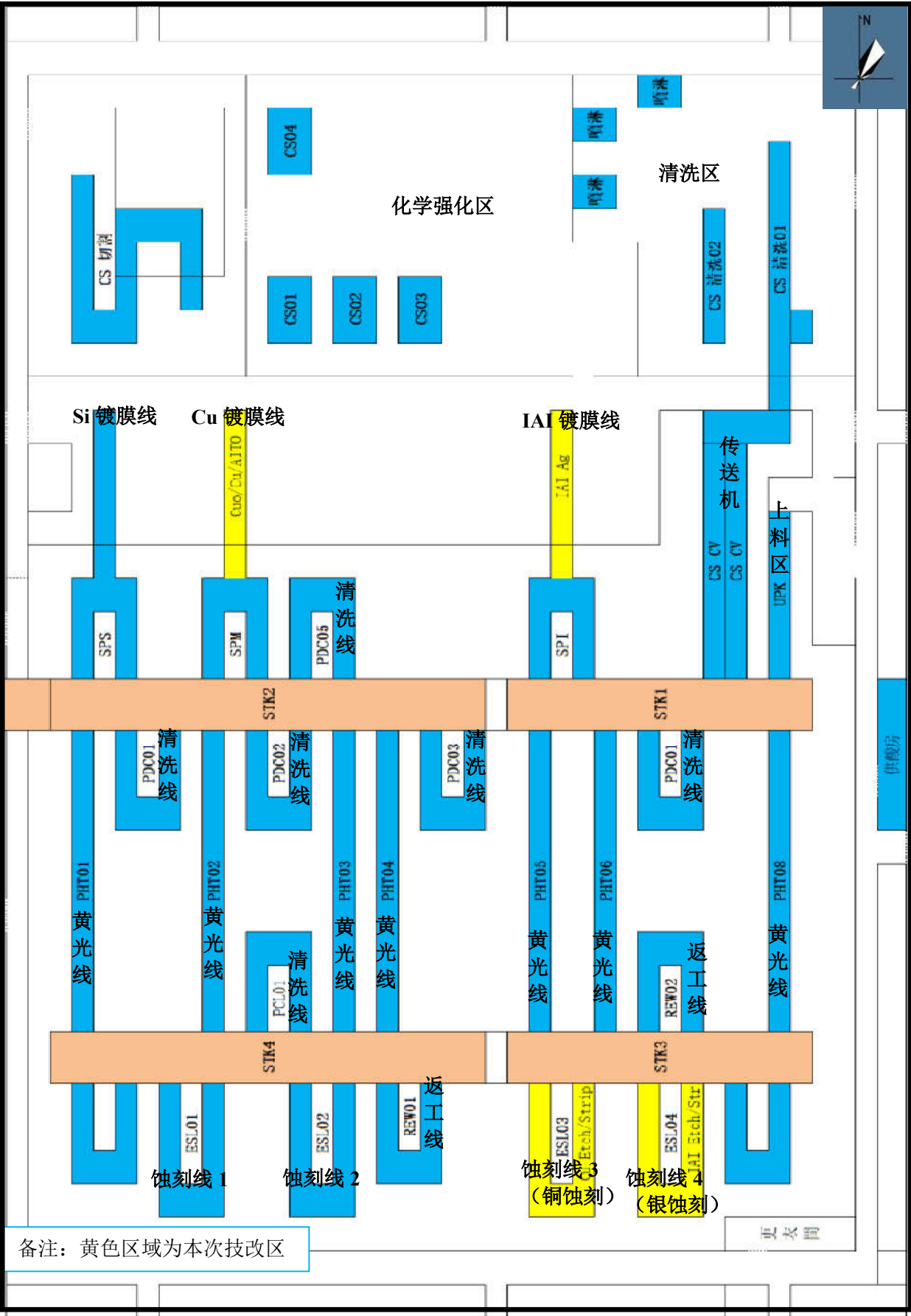
附图 5 车间平面布置图（厂房 A）
